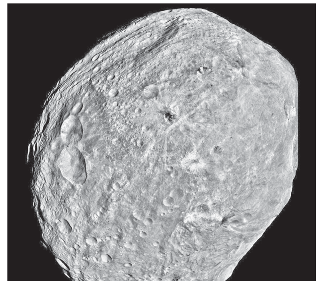
Астероид Веста. Снимок аппарата Dawn NASA с расстояния 5200 км 2011 год
