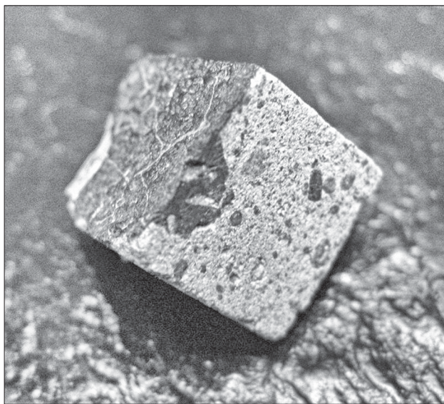
Метеорит Павловка
